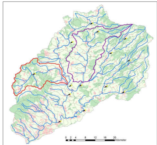
Abbildung 1: Gliederung (Teilgebiete, Hauptfließgewässer und Landnutzung) des Einzugsgebiets im Gesamtmodell mit Pegelstationen (Detailgebiet Usa – rot umrandet; Detailgebiet Horloff – violett umrandet)
