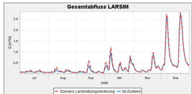
Abbildung 3: Beispielhafte Darstellung des Szenarios Landnutzungsänderung (Erhöhung des besiedelten Flächenanteils, Reduktion der Ackerfläche) auf den Abfluss mit dem Wasserhaushaltsmodell LARSIM
